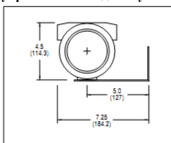
Пластины крепления блока управления – Вид сбоку
