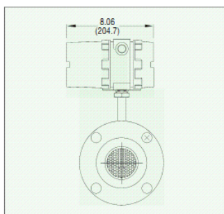
Фланец DN – Вид сбоку (E2)
