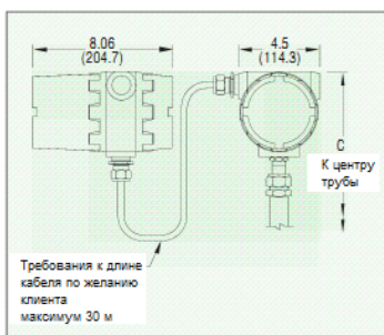
Клеммная коробка, соединенная с блоком управления – Вид спереди (E4)
